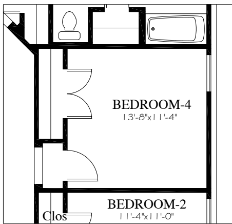
OPTIONAL BEDROOM-4
